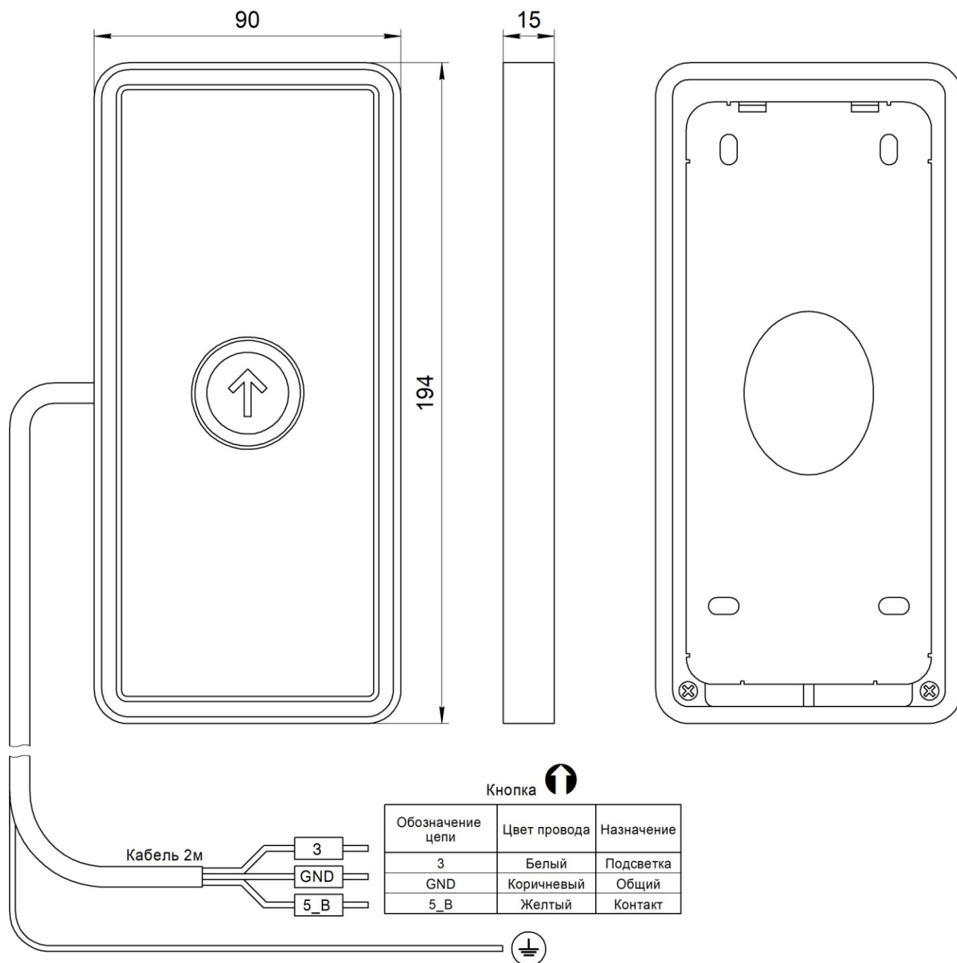
Рис.1 Внешний вид и габаритные размеры Вызывного поста ОБСИДИАН НШЕК.468381.216
